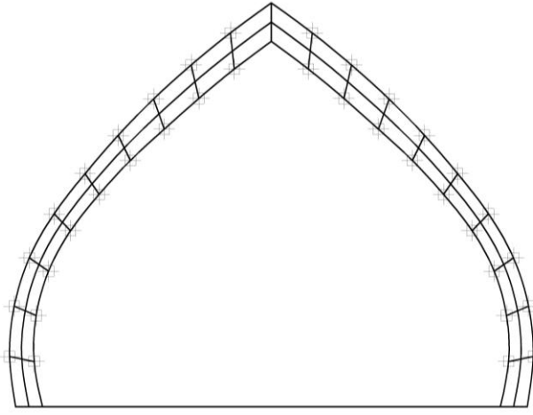
شكل (14) رسم متوسط جديد بين متوسطي المسقطين الافقي والعمودي المصدر : الباحث
