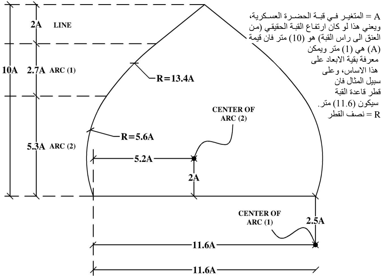
شكل (7) قبة الحضرة العسكرية
