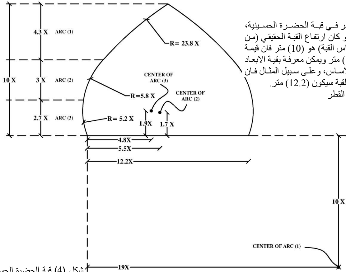
شكل (4) قبة الحضرة الحسينية
