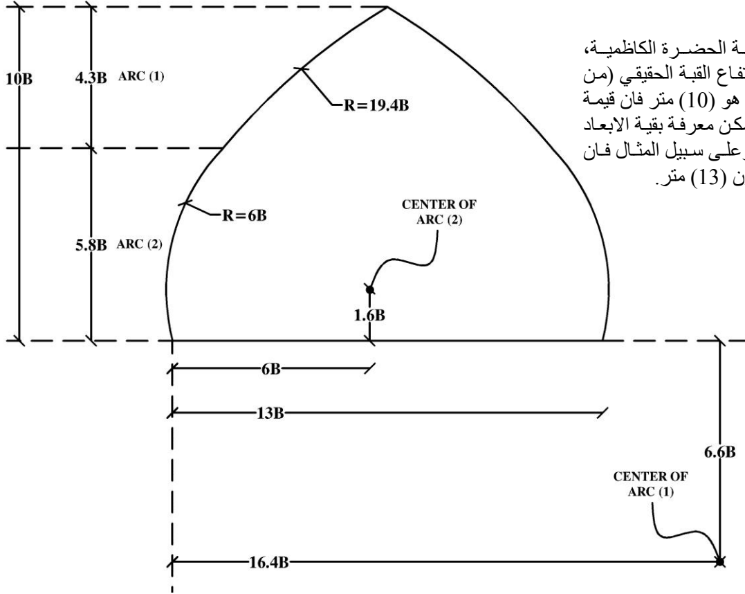
شكل (6) قبة الحضرة الكاظمية
