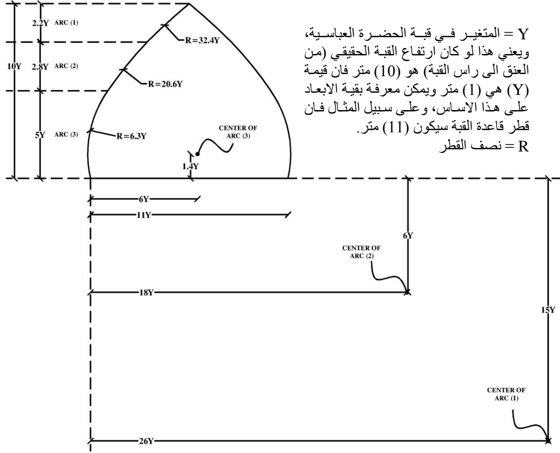
شكل (5) قبة الحضرة العباسية
