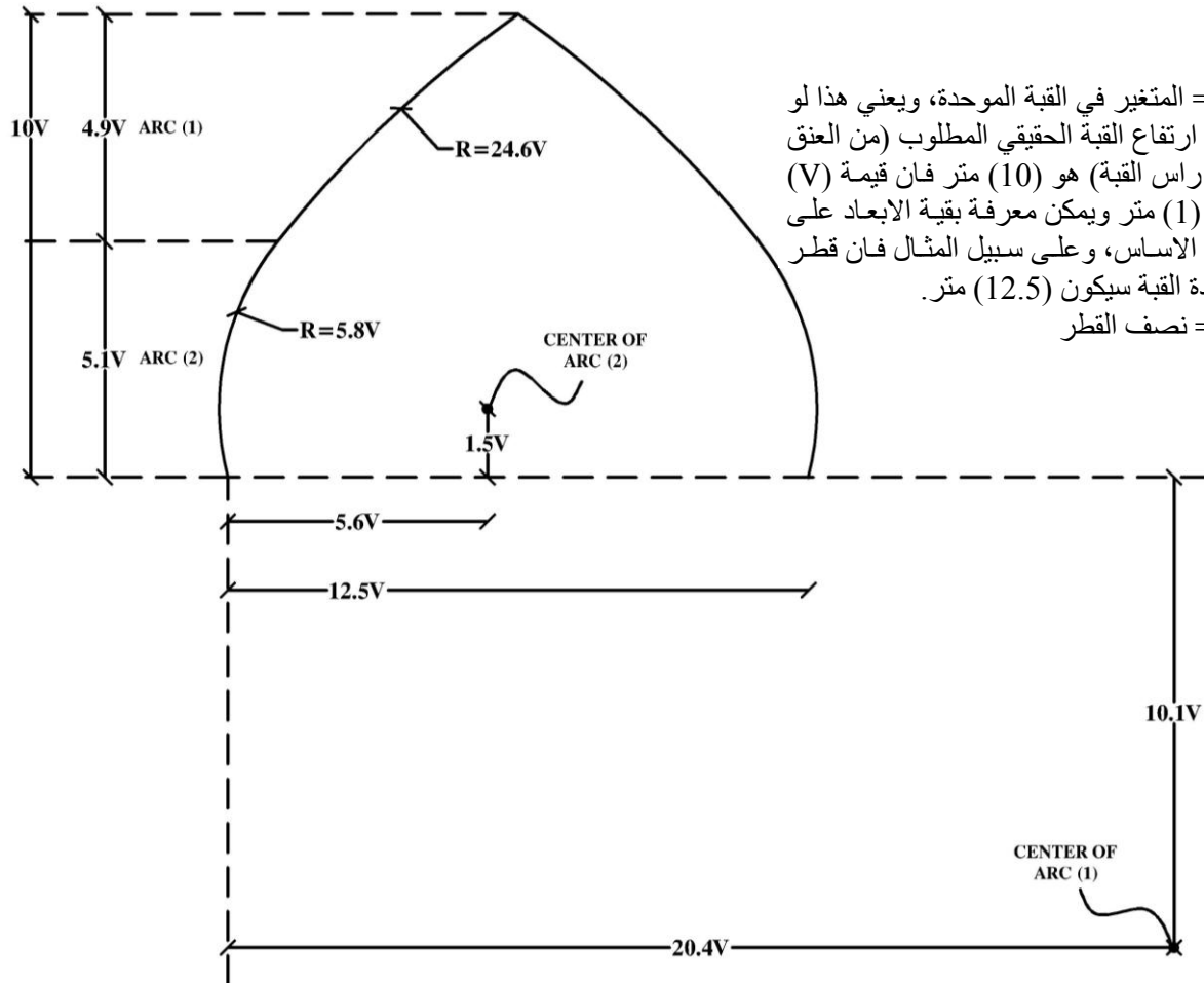
شكل (15) ابعاد القبة الموحدة
